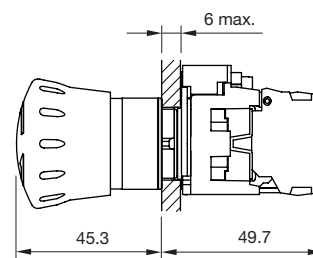
Pilzdrucktaste
