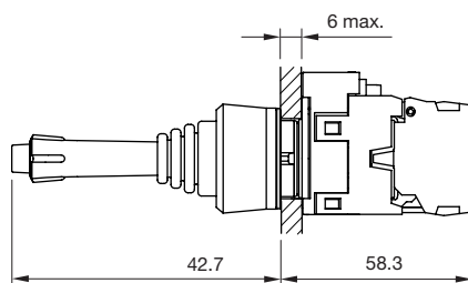
Koordinatenschalter
