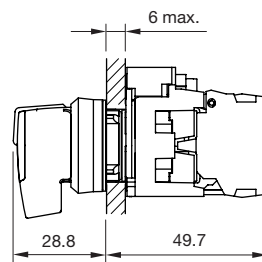
Wahlschalter langer Hebel
