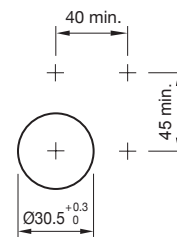
Einbauöffnungen flache Bauform
