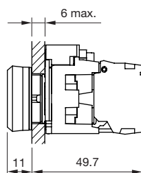
Abmessungen erhabene Bauform Leuchtmelder
