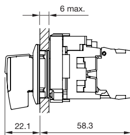
Wahlschalter
