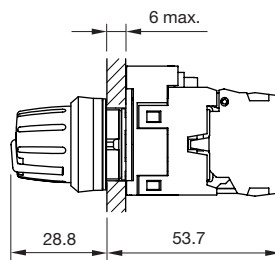
Wahlschalter runder Hebel
