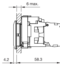
Abmessungen flache Bauform Leuchtmelder/Drucktaste
