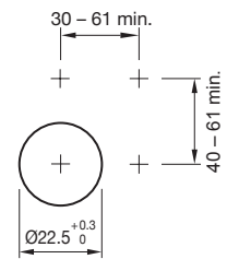
Einbauöffnungen erhabene Bauform
