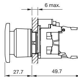
Pilzdrucktaste
