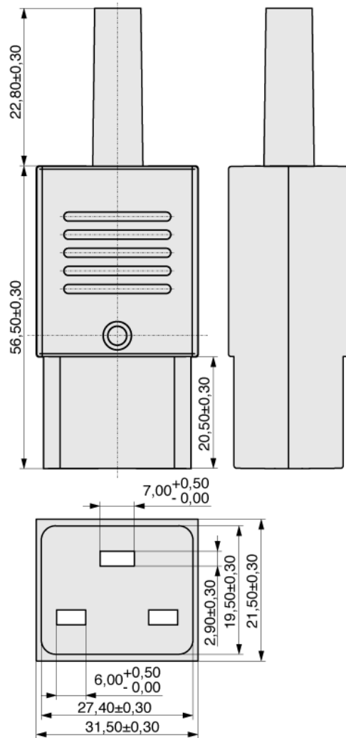
Wiederanschließbare Kabelbuchse
