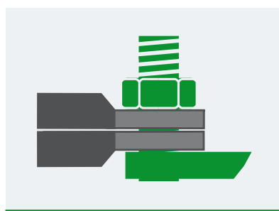
Připojení kabelového oka na svorkovnice
