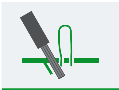
Připojení pružinovými svorkami
