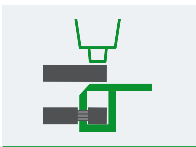
Připojení systémem ADO
